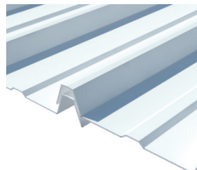
Traslapo lateral
