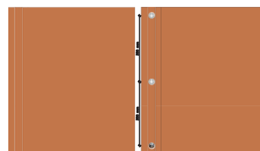
PLANTA - Arkowood wallpanel exterior
